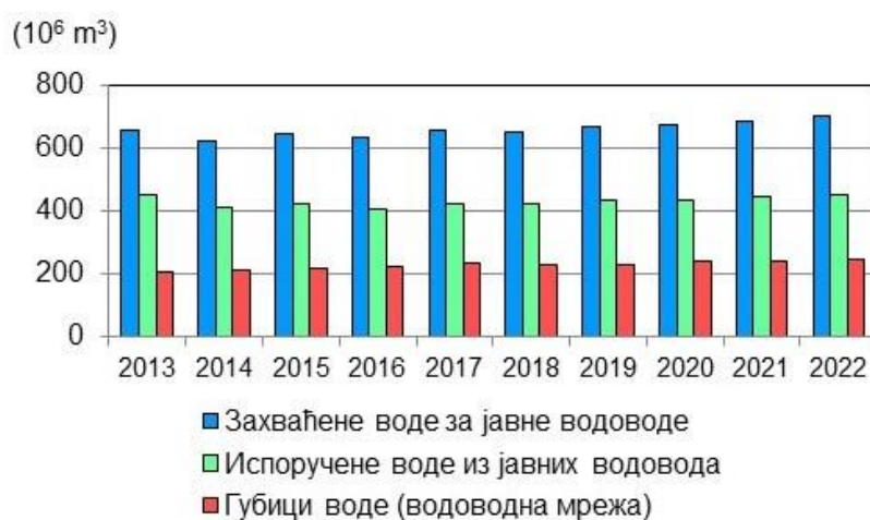
Слика 3.5.28. Ефикасност коришћења вода у водоводима Републике Србије (2013-2022. године)
