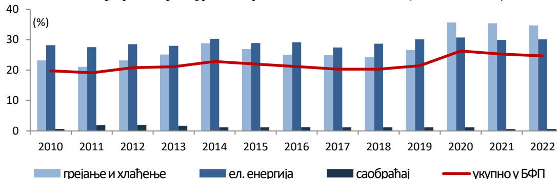
Слика 3.5.51. Удео ОИЕ у бруто финалној потрошњи енергије у Републици Србији
