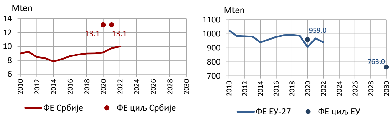
Слика 3.4.5. Потрошња ФЕ и циљеви потрошње у Републици Србији и Европској унији
